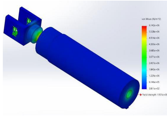
Fig. 8. Von Mises Stress in CR with Al 5056
