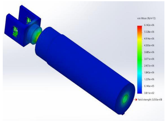
Fig. 14. Von Mises Stress in CR with Al 7075
